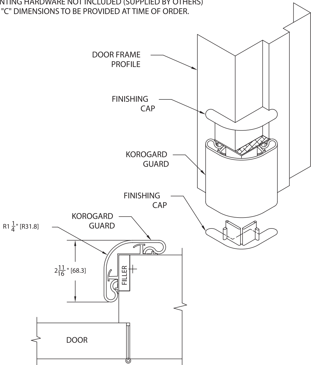
F360, DOOR FRAME GUARD SCALE: 1:2
